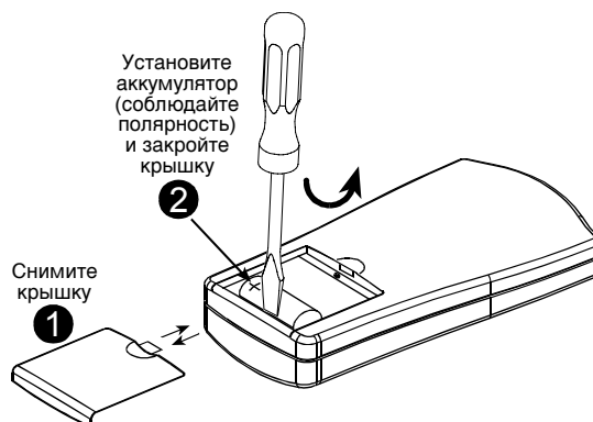
Рисунок 3 – Замена аккумулятора
