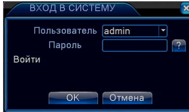
Рис. 3.1 Вход в систему
