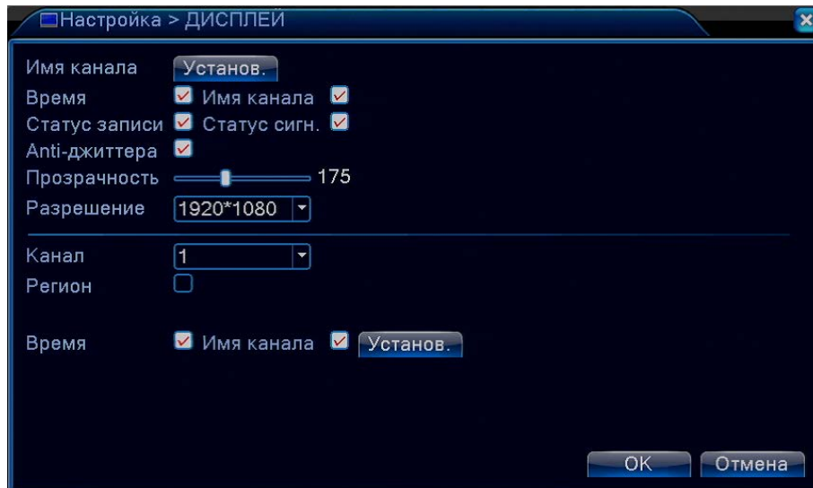
Рис.4.37 Экран графического интерфейса
