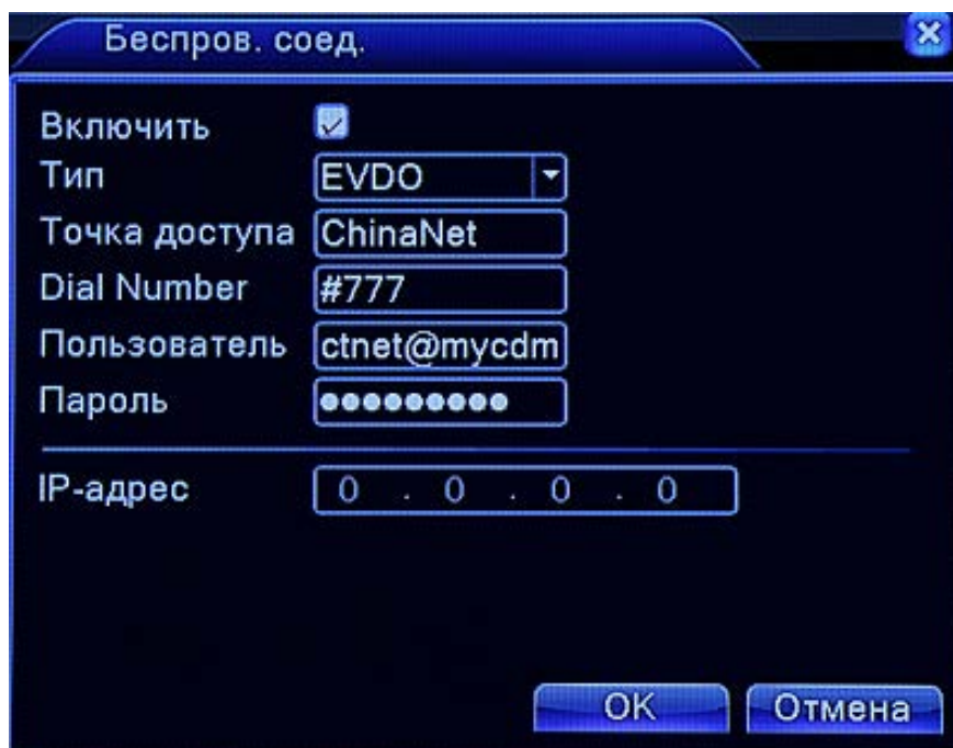
Рис. 4.32 Настройки беспроводного соединения
