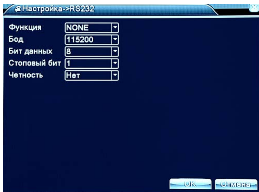
Рис. 4.39 Настройка RS232
