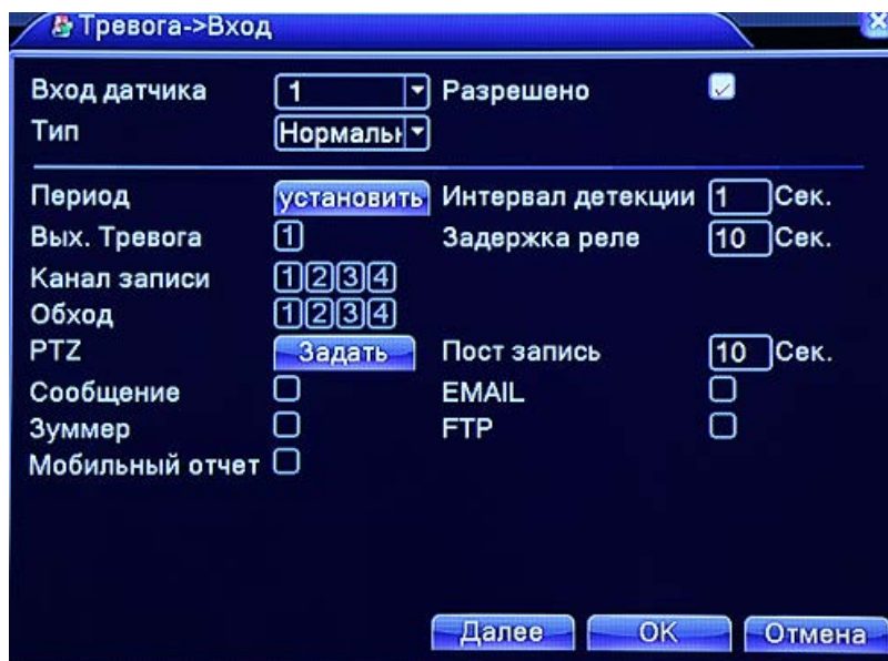
Рис. 4.10 Сигнал тревоги
