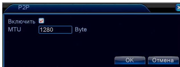
Рис. 4.36 Настройка WiFi
