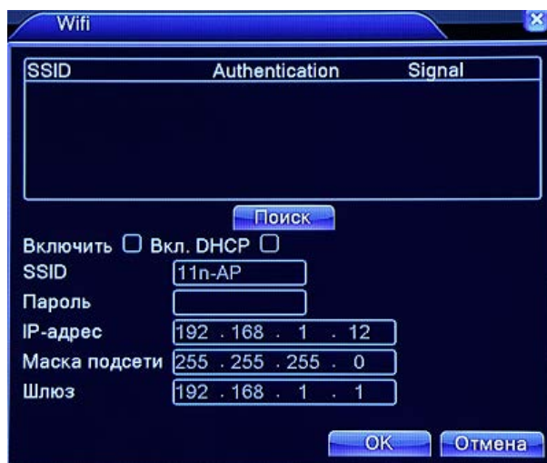
Рис. 4.34 Настройка Wi-Fi
