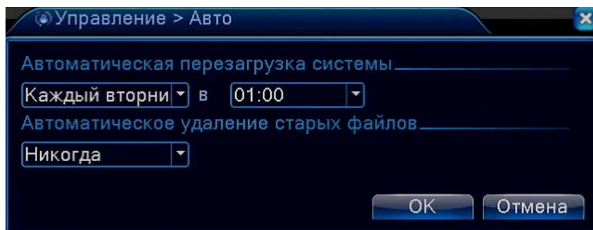
Рис 4.49 Автоматические настройки
