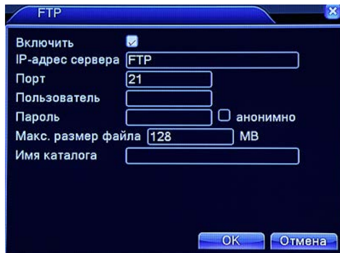
Рис. 4.29 Настройки FTP
