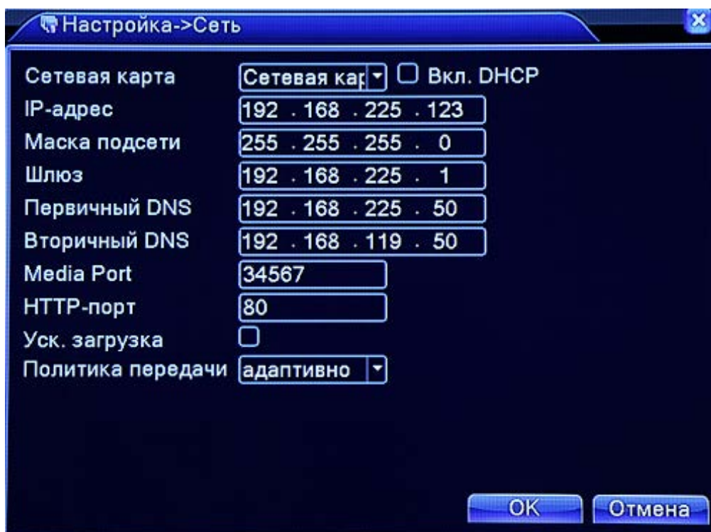
Рис. 4.22 Сетевое соединение
