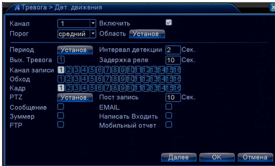
Рис 4.4 Обнаружение движения
