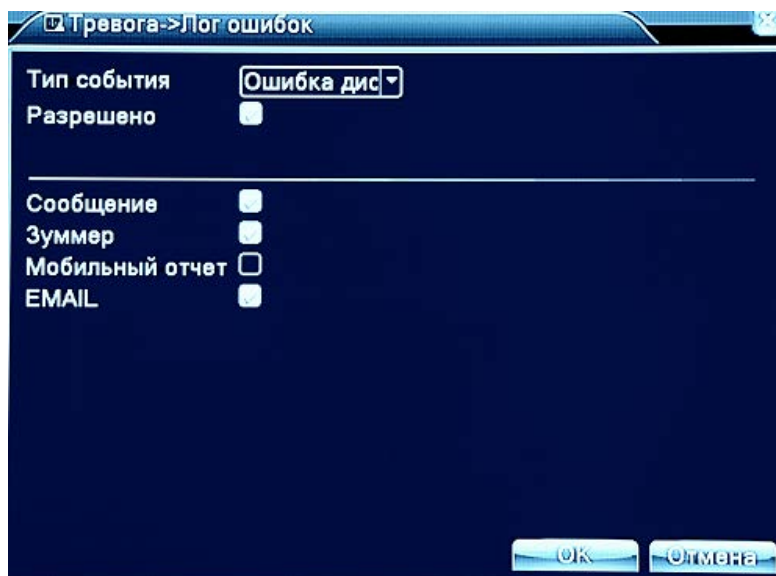
Рис 4.11 Диагностика неисправностей
