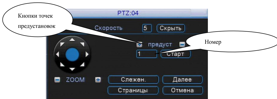
Рис. 3.11 Настройка предустановок
