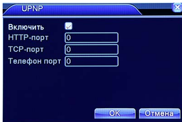
Рис. 4.33 UPNP
