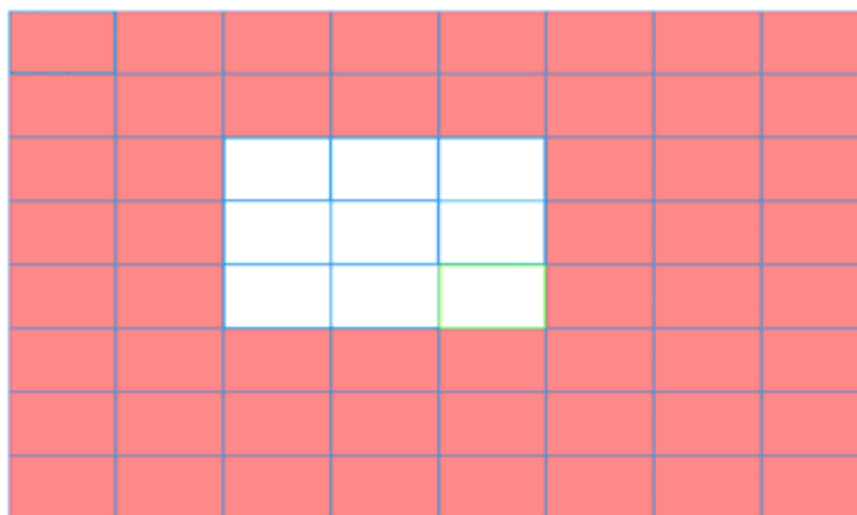
Рис 4.5 Область
