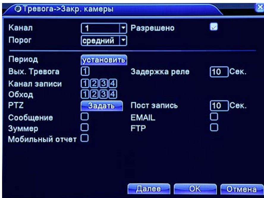
Рис 4.8 Закрытие камеры
