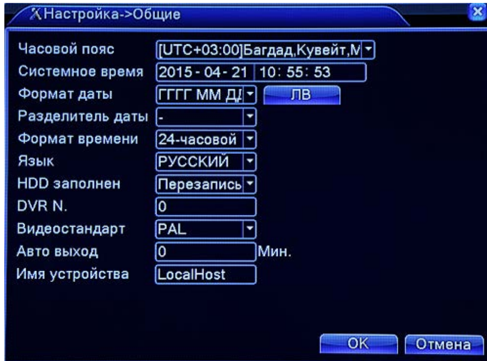
Рис. 4.19 Общие настройки
