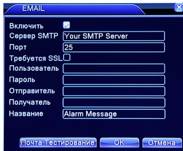
Рис. 4.26 EMAIL
