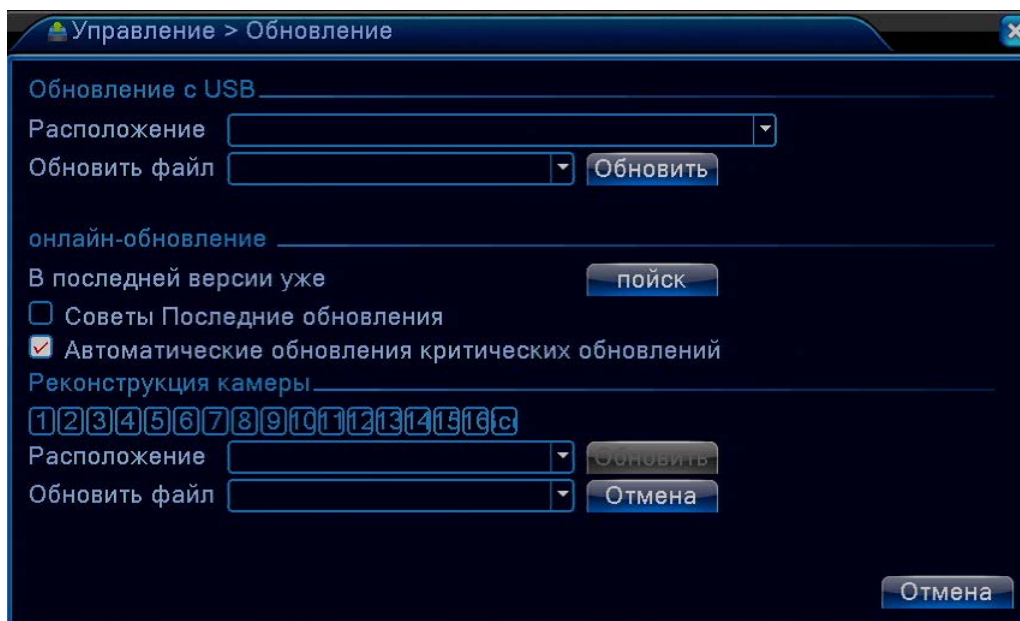
Рис. 4.51 Обновление ПО
