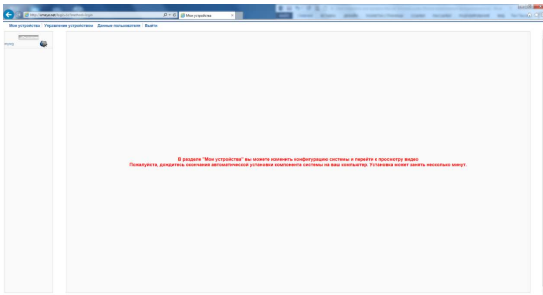
Рис. 5.3 Начальное окно
