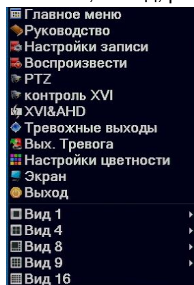
Рис 3.2 Контекстное меню
