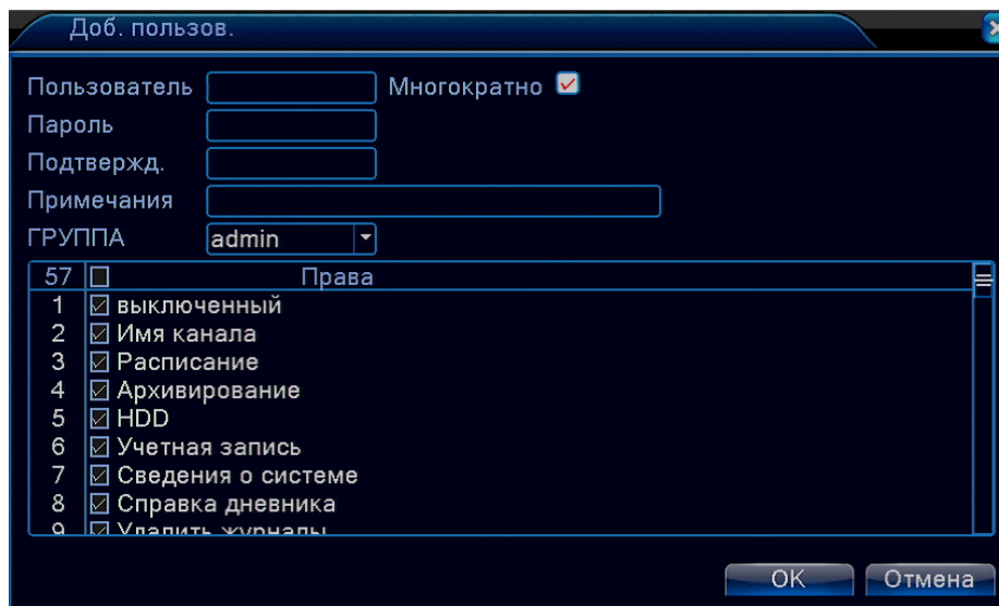
Рис 4.44 Добавление пользователя
