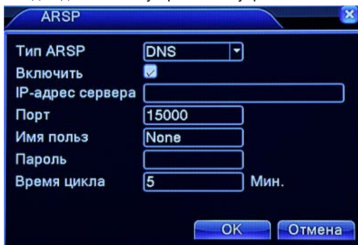
Рис. 4.30 ARSP
