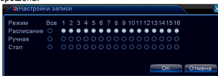
Рис 3.8 Режим записи
