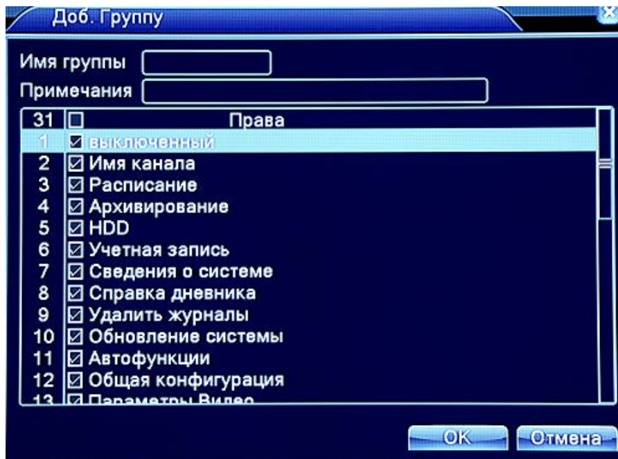
Рис 4.45 Добавление группы
