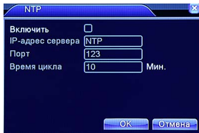
Рис. 4.25 NTP сервер
