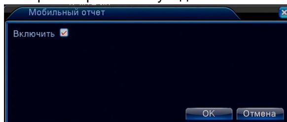
Рис. 4.36 Мобильный отчет
