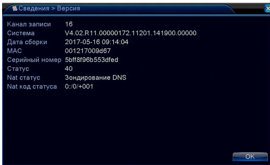
Рис 4.56 Версия ПО
