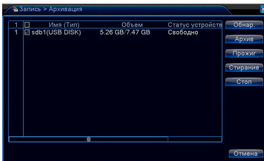
Рис. 4.3. Копирование
