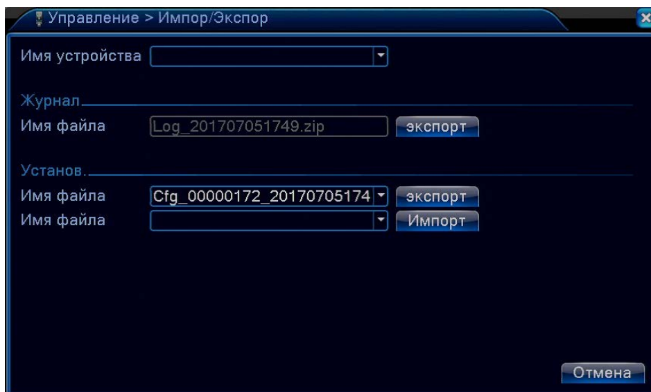
Рис 4.53 Импорт/экспорт
