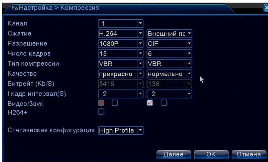
Рис. 4.21 Настройки кодирования
