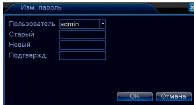
Рис. 4.43 Изменение пароля
