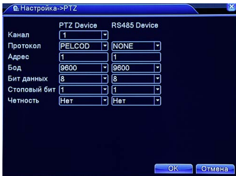
Рис. 4.38 Настройка PTZ
