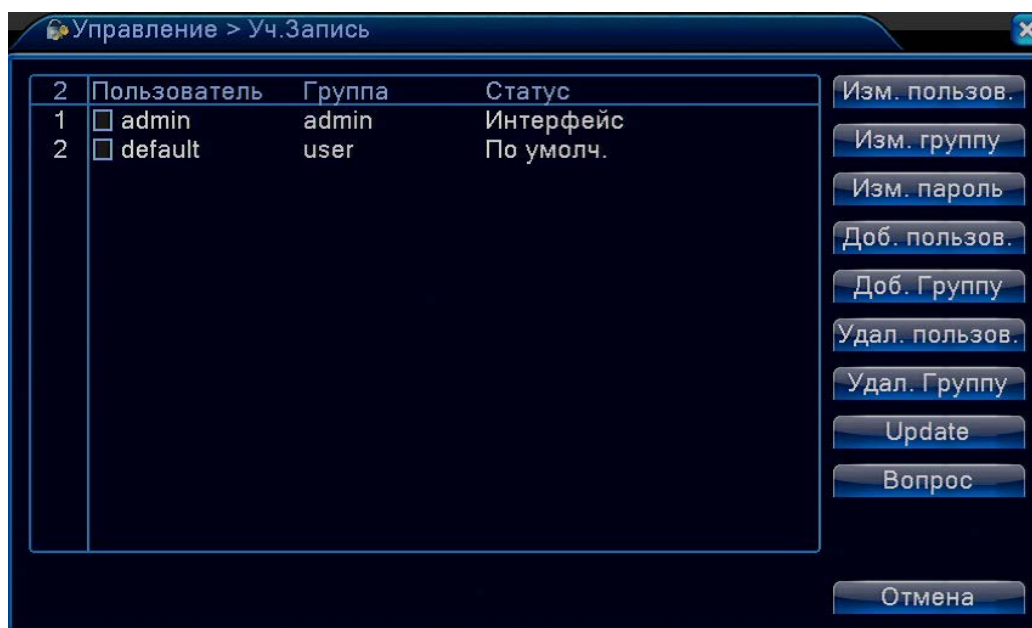
Рис. 4.42 Учетные записи
