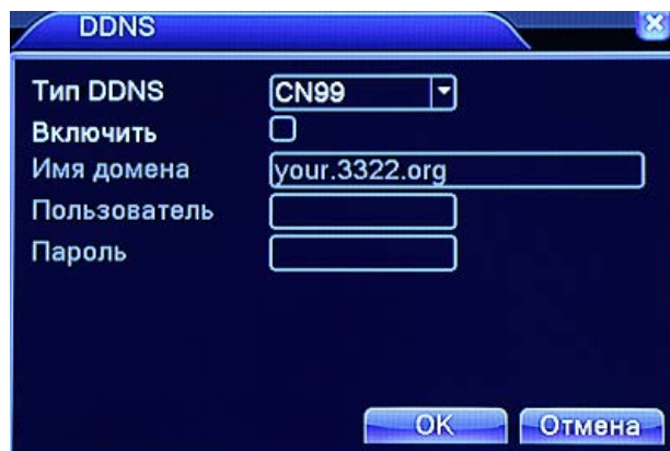
Рис. 4.28 Установка DDNS
