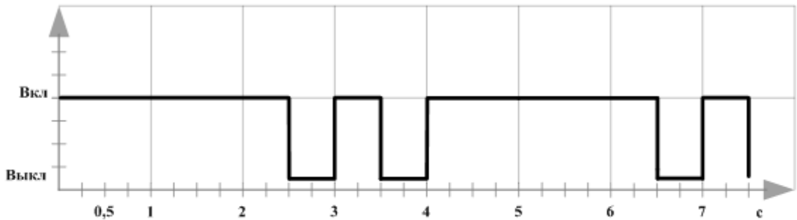
Рис. 11.5. Индикация режима На охране со шлейфом в состоянии Тревога и режима На охране с аварией
