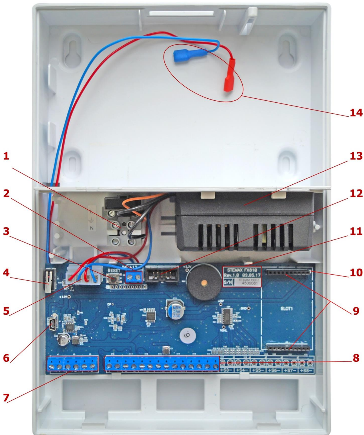
Рис. 11.1. Вид контроллера со снятой крышкой
